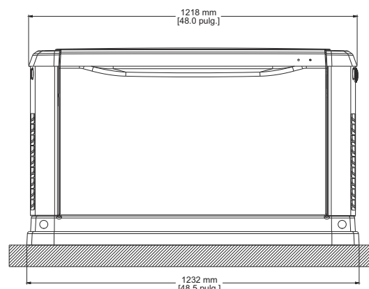
VISTA DELANTERA
